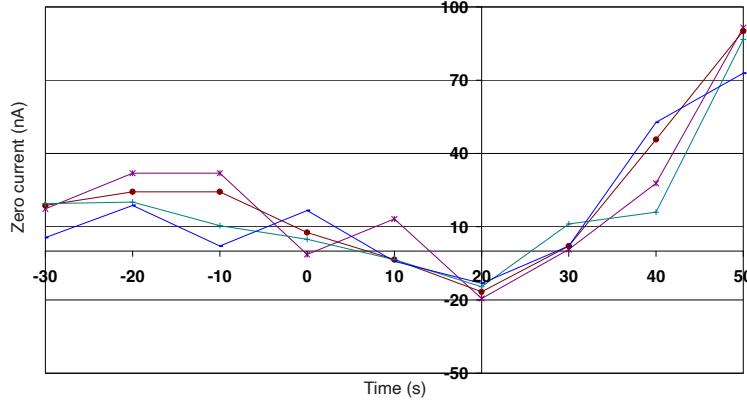
图2 零点温度特性（未修正）
