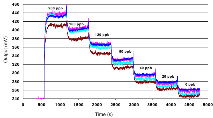
图3 0~200ppb的线性度
