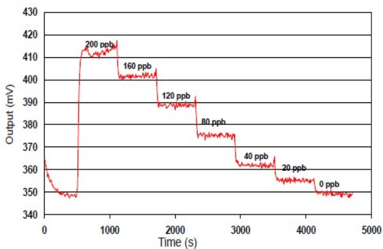
图3 对200ppb SO 2 的反应
