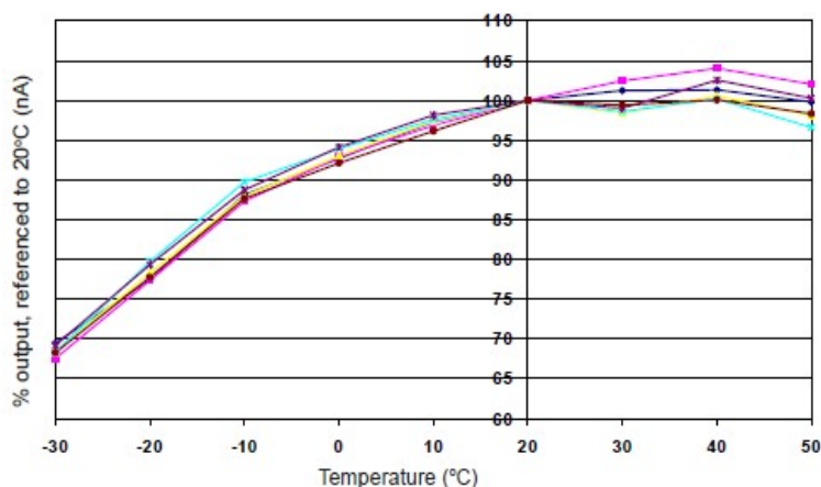
图1 灵敏度温度特性
